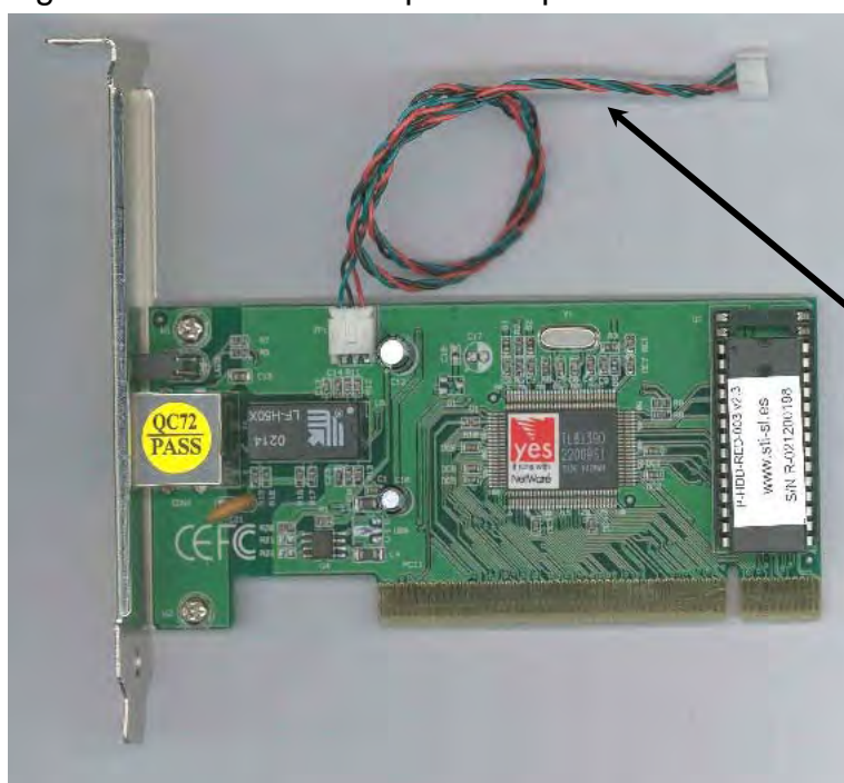
Cable WOL
